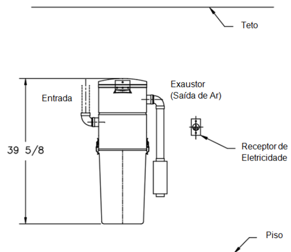
VISTA FRONTAL MODELO FC570
