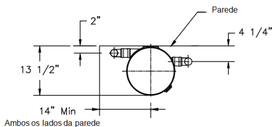
VISTA SUPERIOR MODELO FC570
